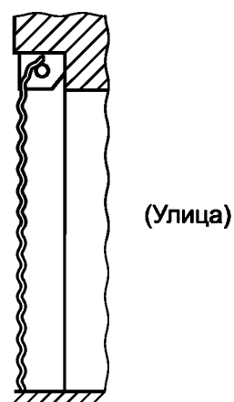
Полотно вне проема, устройство намотки с защитным коробом внутри стенового проема
