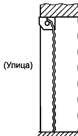
Полотно в проеме, устройство намотки с защитным коробом снаружи
