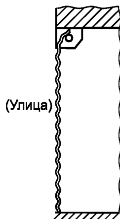
Полотно в проеме, устройство намотки с защитным коробом внутри стенового проема
