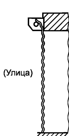
Полотно вне проема, устройство намотки с защитным коробом снаружи
