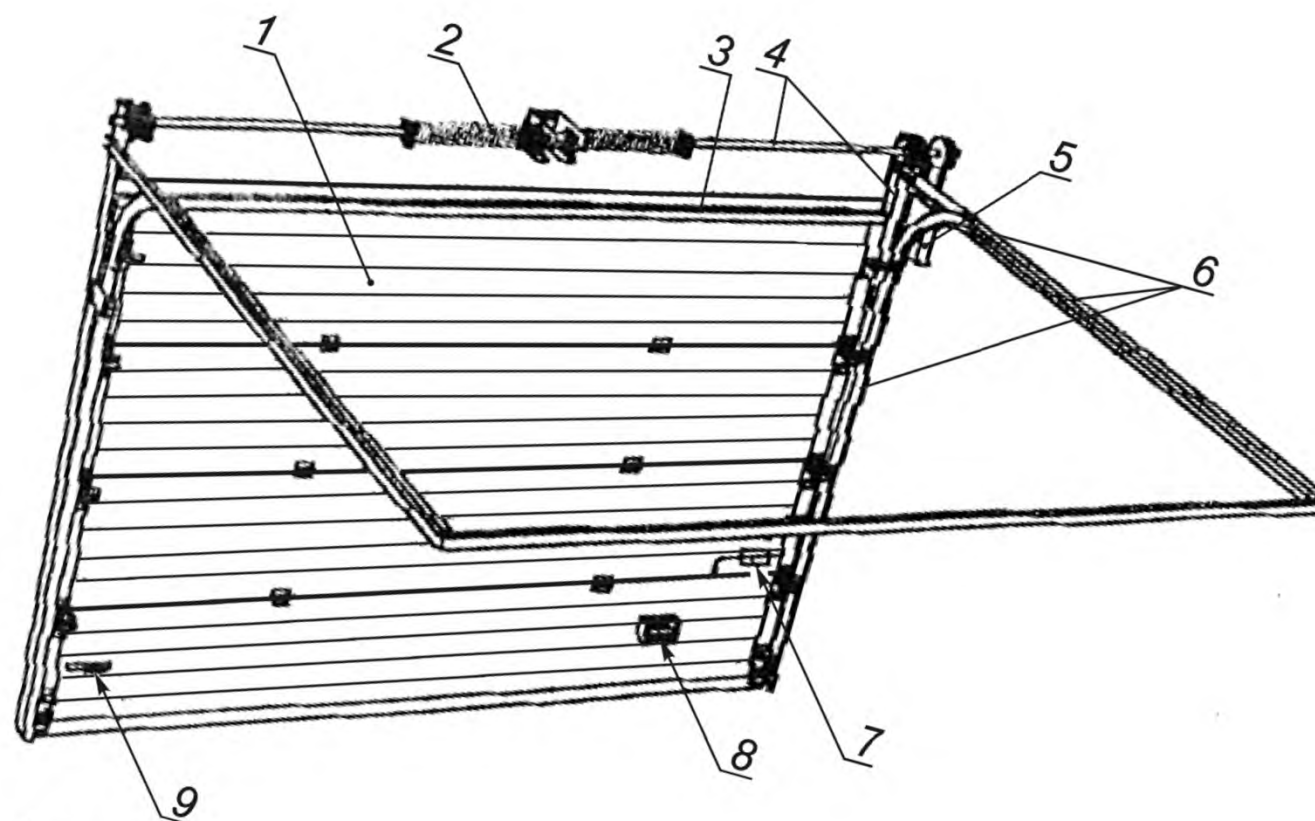
1 — полотно ворот; 2 — система уравнивания полотна; 3 — уплотнитель; 4 — элементы обрамления проема; 5 — привод; 6 — направляющие профили; 7 — задвижка; 8 — ручка; 9 — запирающее устройство Рисунок Б.4 — Подъемно-секционные ворота
